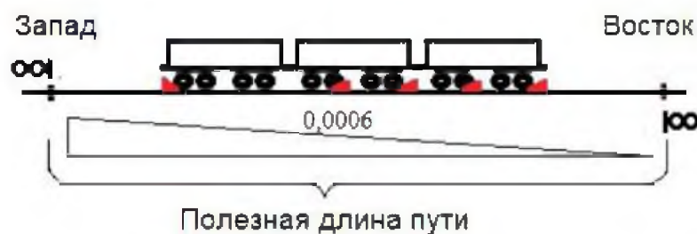
Рис. 1. Схема укладки тормозных башмаков под вагоны
