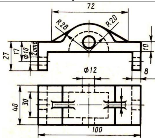
Корпус
