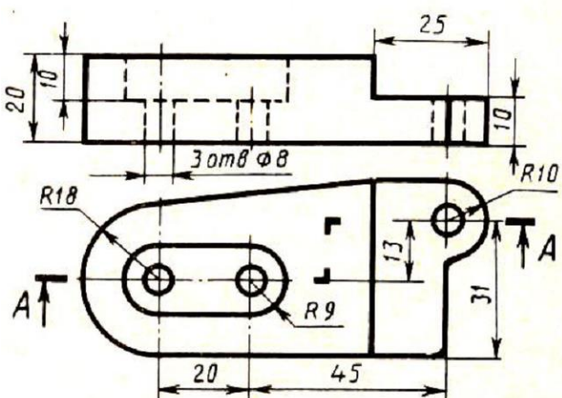
Плита
