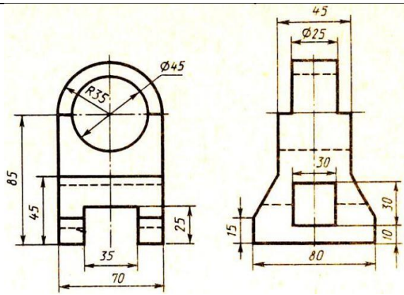
Кронштейн
