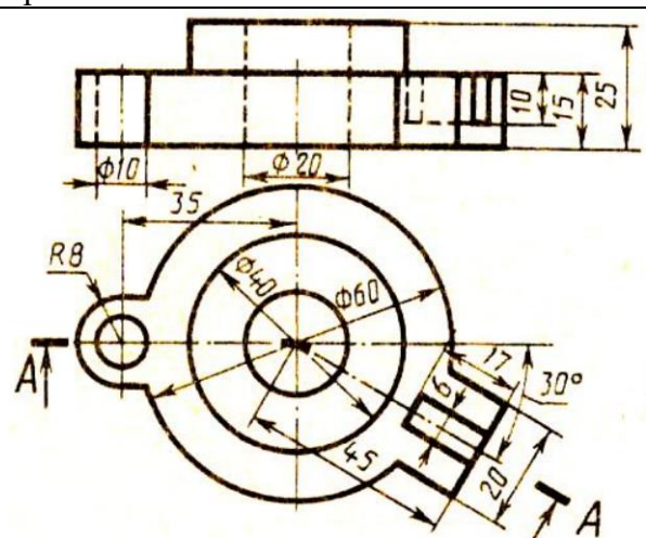
Диск
