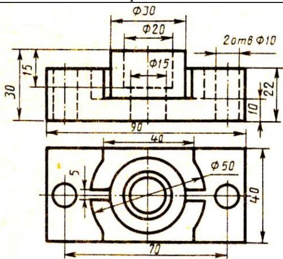
Корпус
