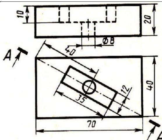
Плита
