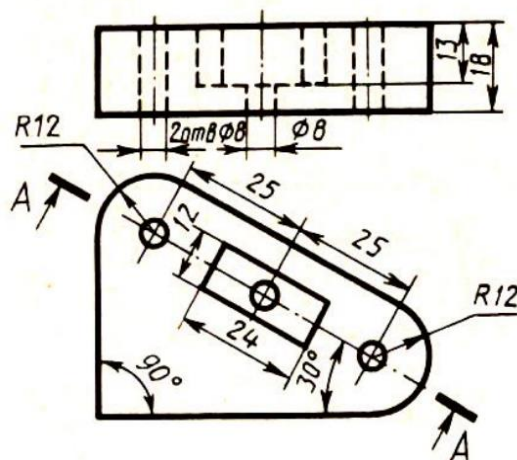
Пластина
