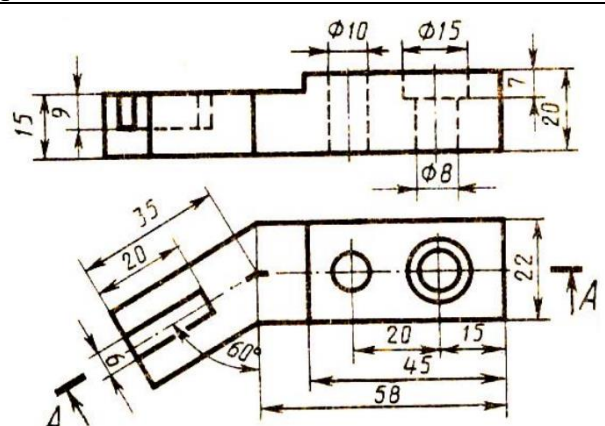
Скоба
