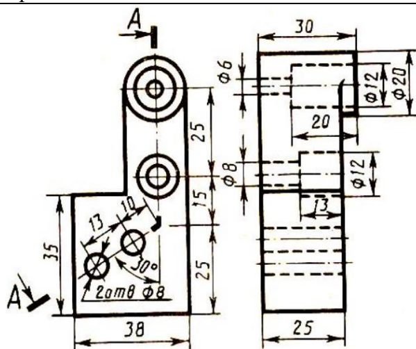
Кронштейн
