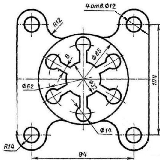
Крышка
