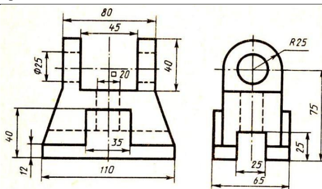
Кронштейн
