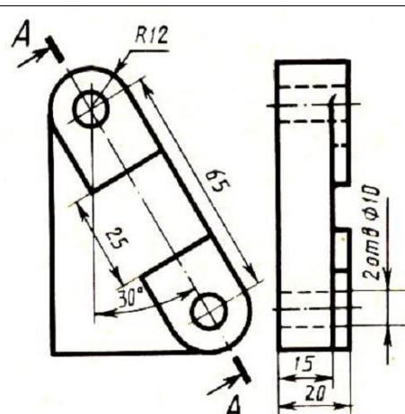
Пластина
