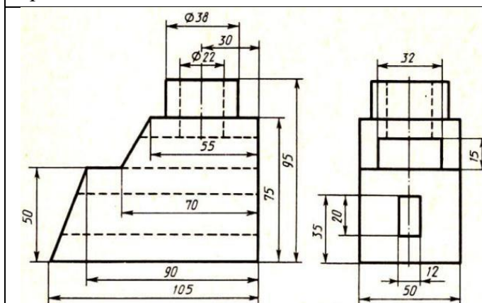
Корпус
