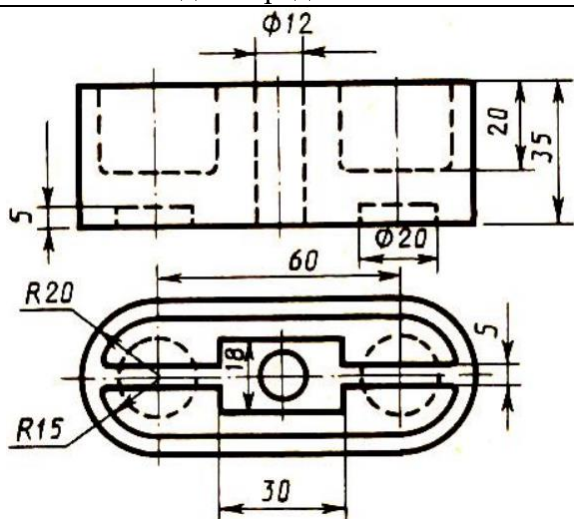
Коробка
