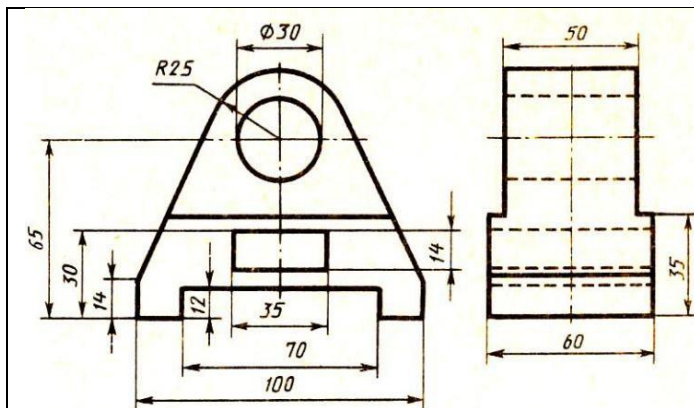
Стойка
