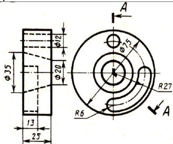
Замок
