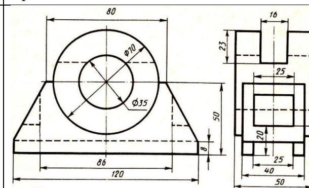
Подшипник
