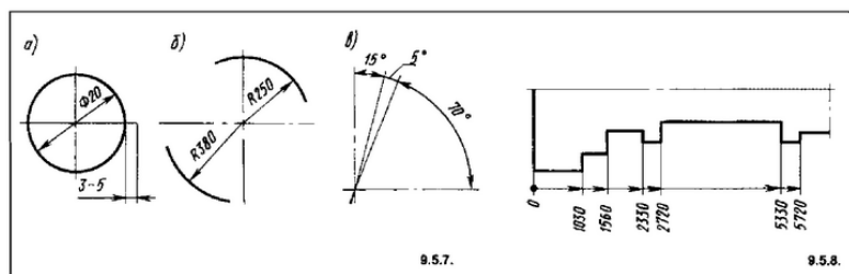
Рисунок 3 Нанесение отметок
