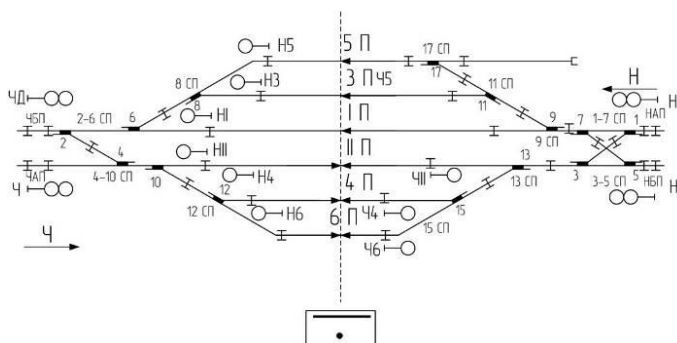
Рисунок 9 Чертеж схемы станции
