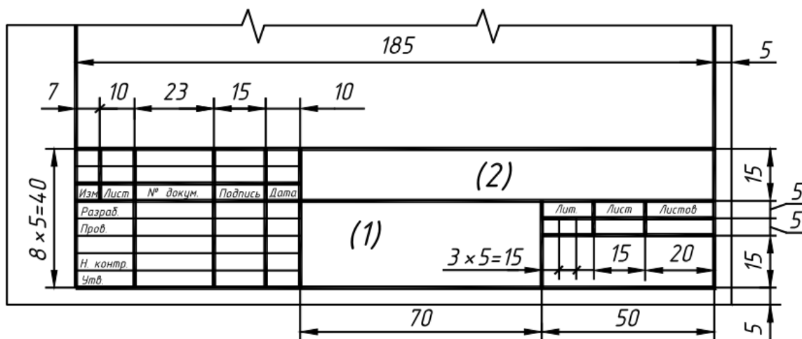
Рисунок 4 Основная надпись (форма 2)
