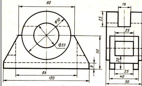
Стойка
