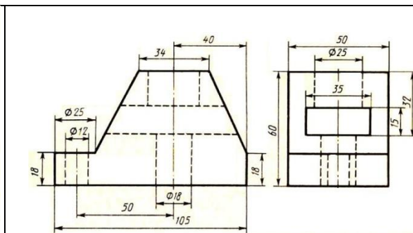
Опора
