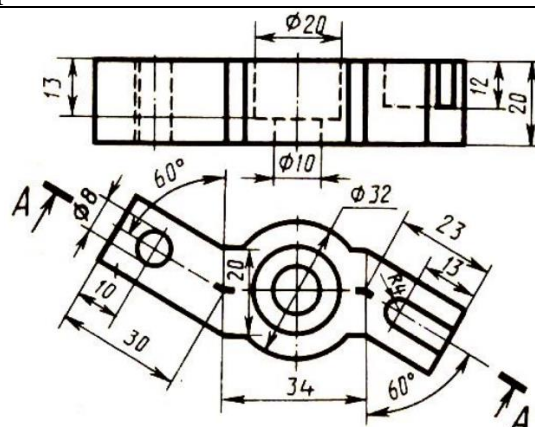
Скоба
