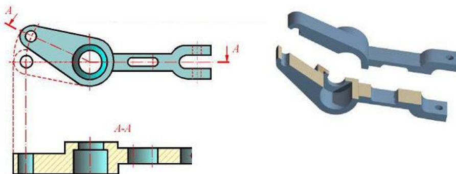
Рисунок 2 Разрез ломаный
