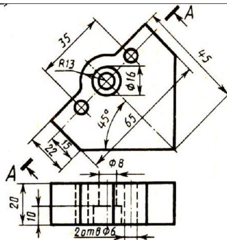
Пластина
