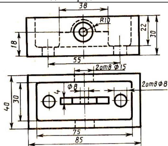
Коробка
