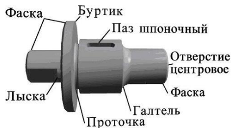
Рисунок 2 - Конструктивные элементы детали
