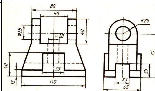
Кронштейн
