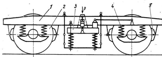
Рисунок 1 Схема тележки КВЗ-ЦНИИ 1
