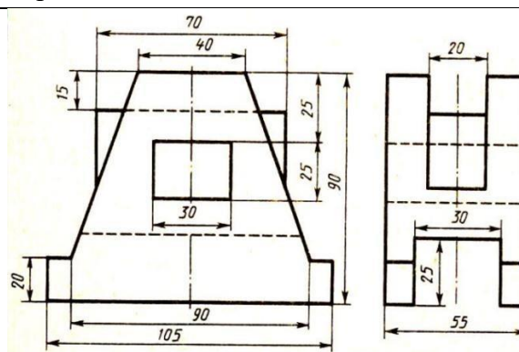
Станина
