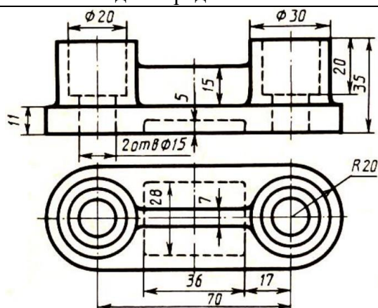
Опора
