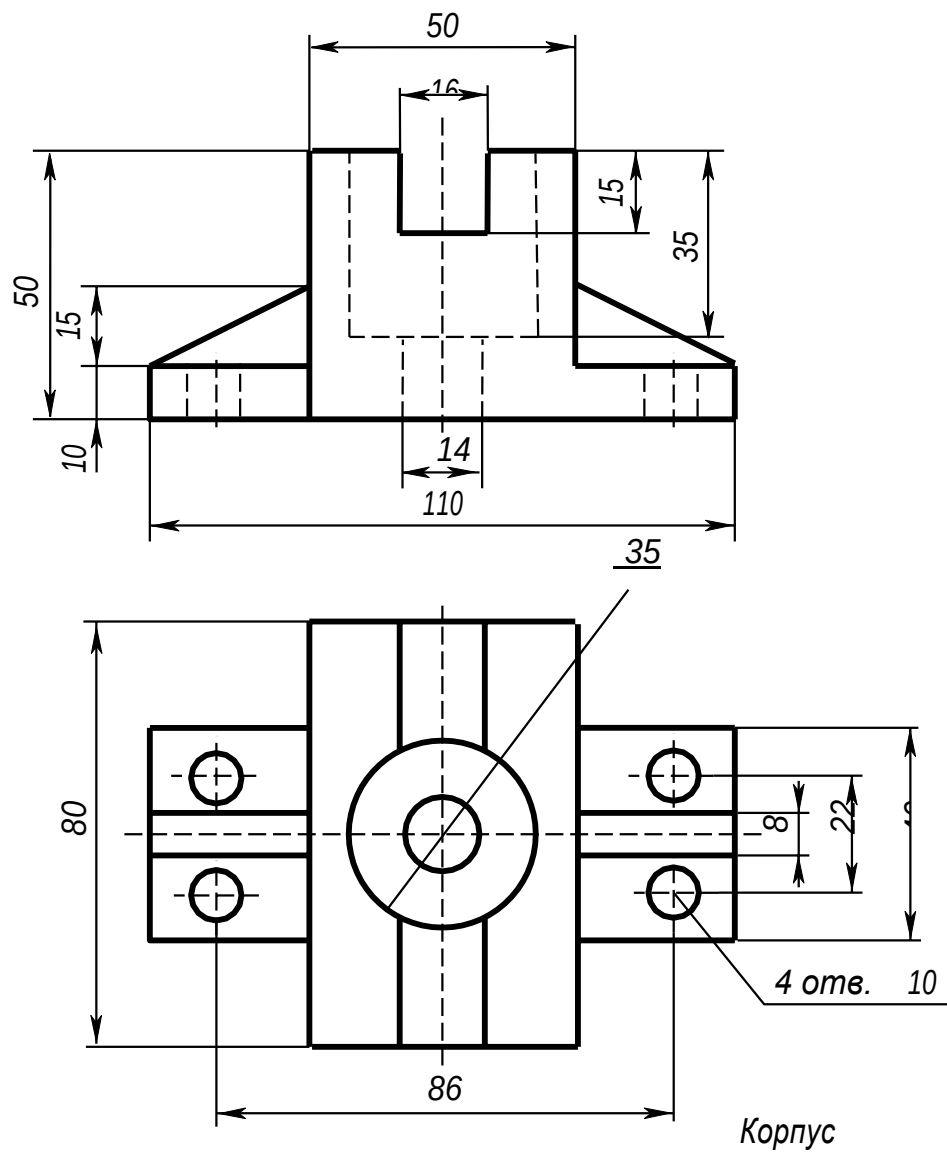
Рисунок 1 Образец задания
