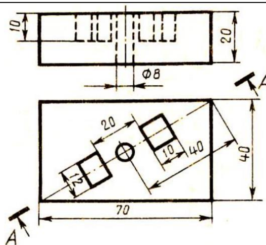
Плита
