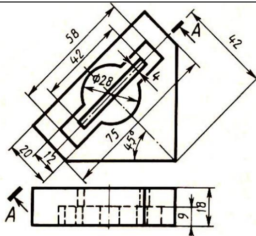
Пластина
