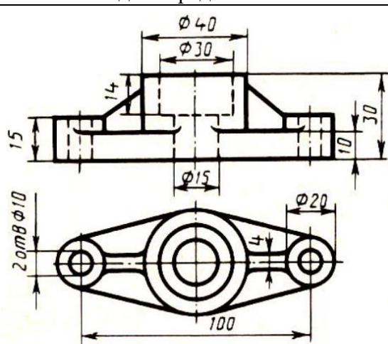
Фланец
