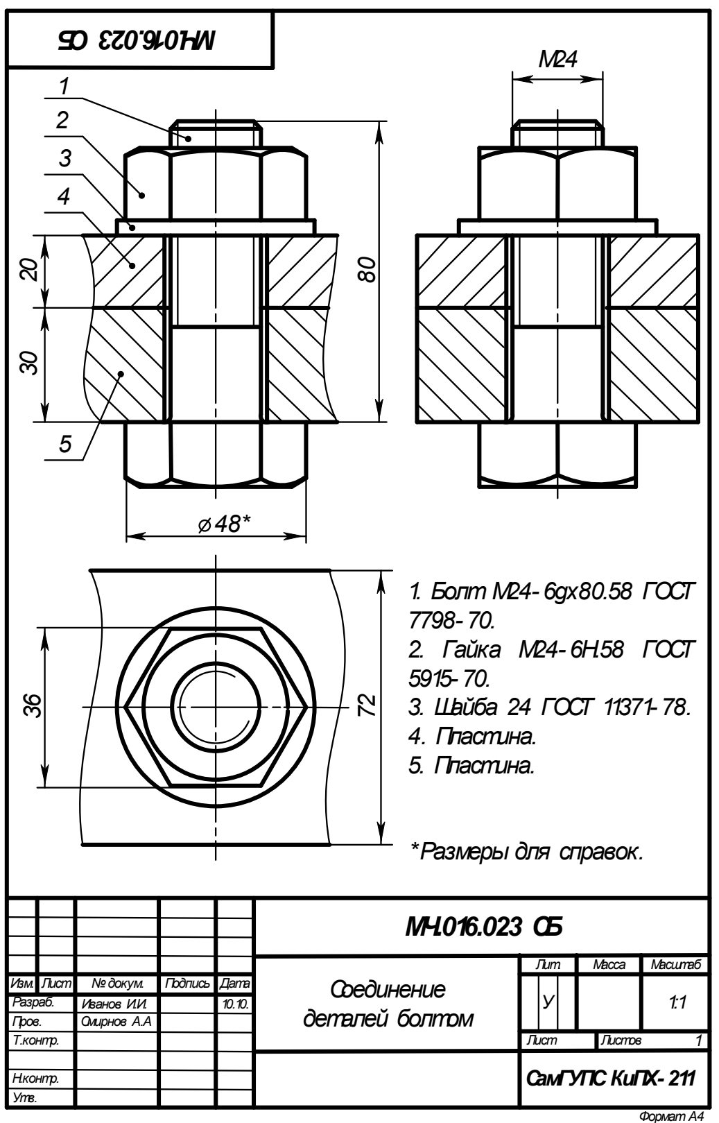
Рисунок 16 Образец выполнения чертежа «Соединение деталей болтом»
