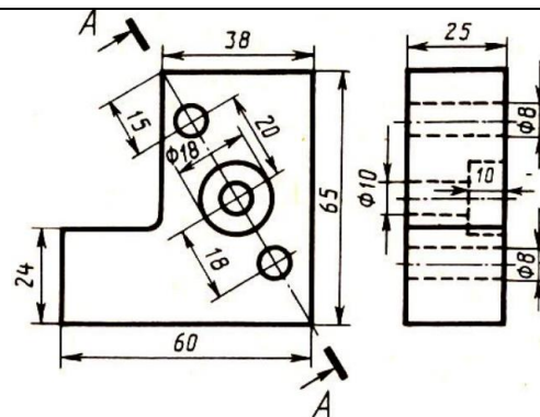
Стойка
