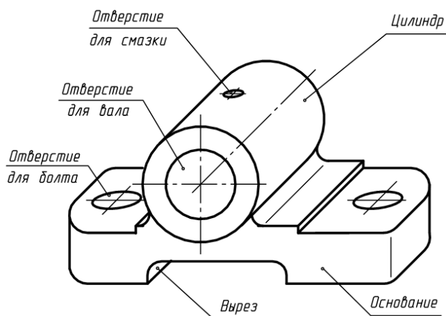
Рисунок 4 Корпус подшипника
