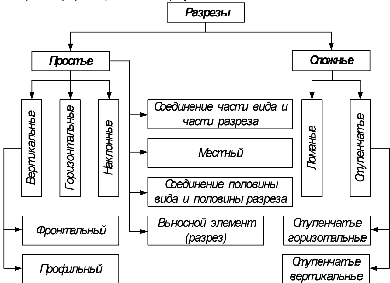
Рисунок 1 Классификация разрезов
