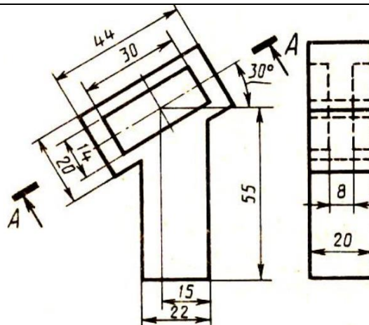
Пластина
