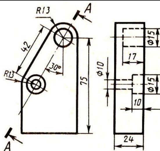
Планка
