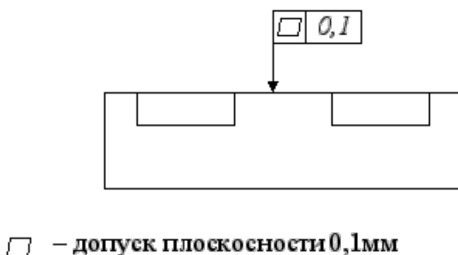
Рисунок 1 Обозначение формы поверхности детали
