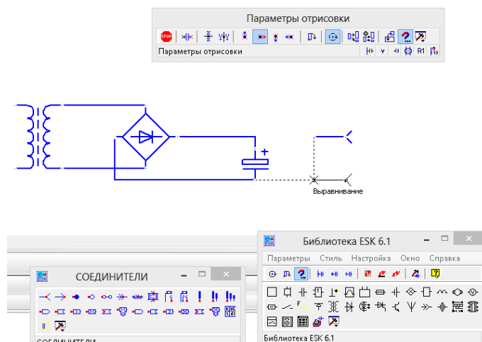
Рисунок 10.9 – Выполнение соединителей
