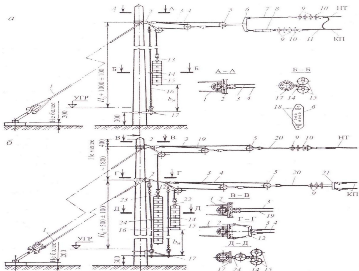
Рис. 1.1. Анкеровка компенсированной цепной контактной подвески переменного (я) и постоянного (б) тока:
