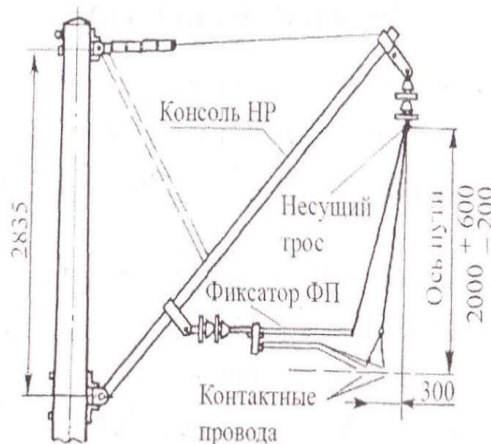
Рис. 1.4. Крепление несущего троса на неизолированной консоли
