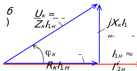
Рис.6. Схема первичной обмотки трансформатора и векторная диаграмма напряжений на ней в режиме КЗ.
