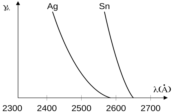
Рис.1.4. Спектральная чувствительность U_{\lambda} фотоэлектрода
