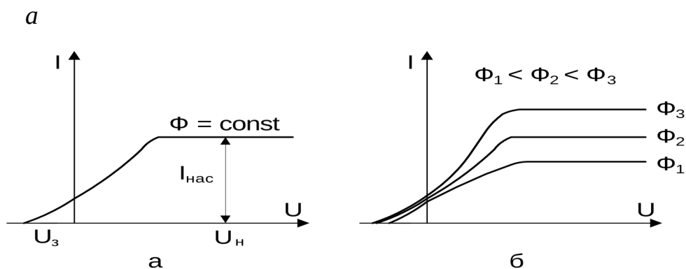
Рис.1.2. Вольтамперные характеристики фотоэлемента
