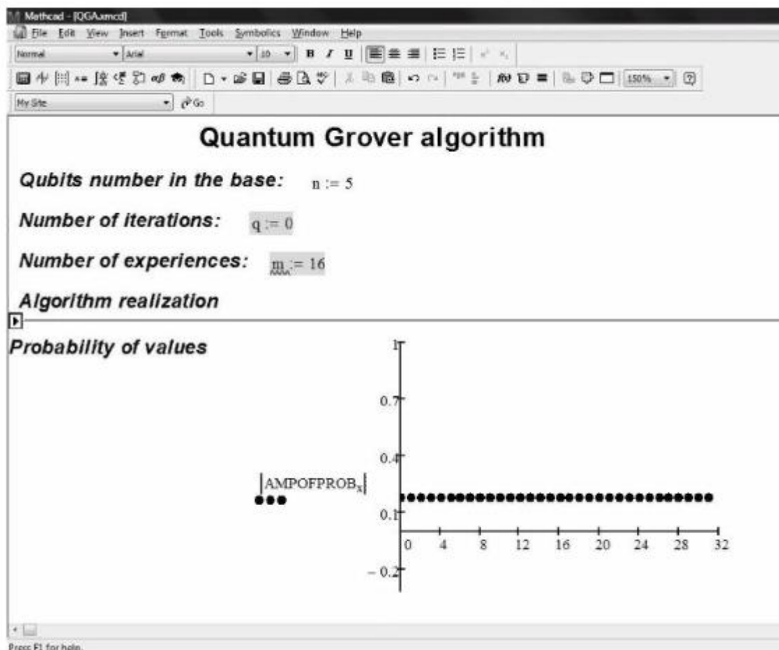
Рис.1. Реализация алгоритма Гровера: распределение амплитуд
