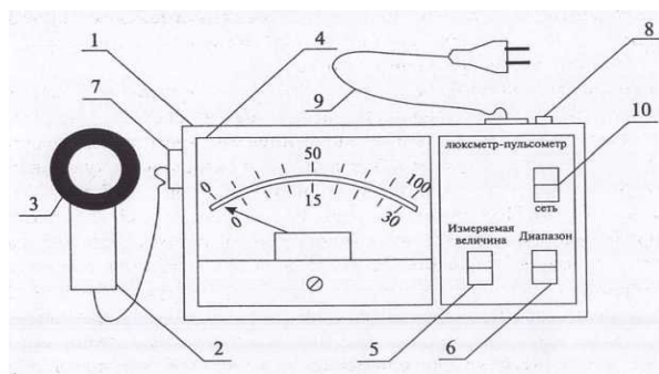
Рис. 2. Внешний вид люксметра-пульсометра «БЖшМ»
