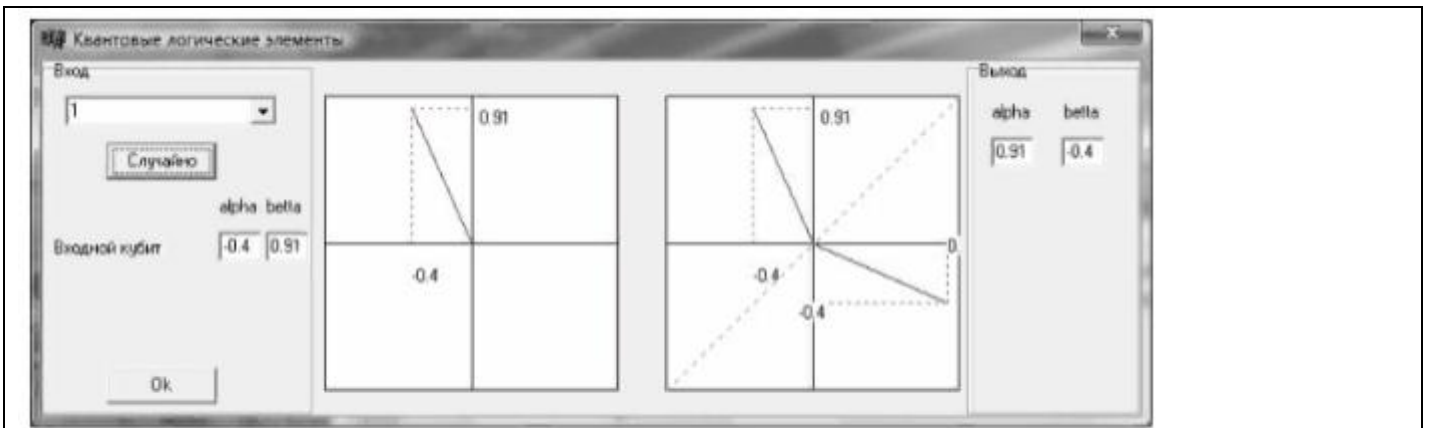
Рис.3. Исследование неизвестного квантового элемента
